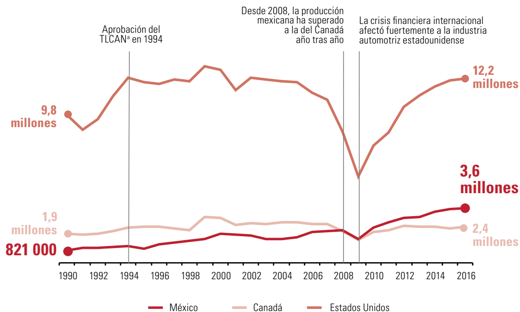
Gráfico III.1 América del Norte: producción de vehículos por país, 1990-2016 (En unidades y porcentajes)
