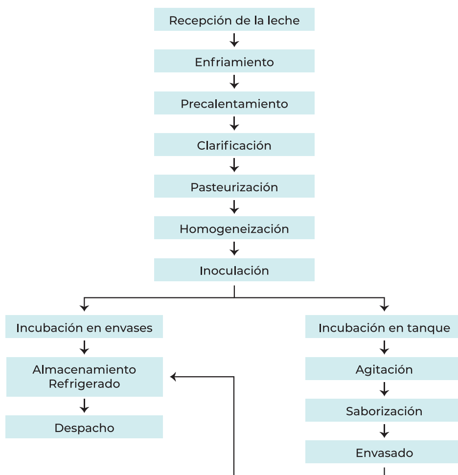
Flujograma 3: Proceso de elaboración de yogurt
