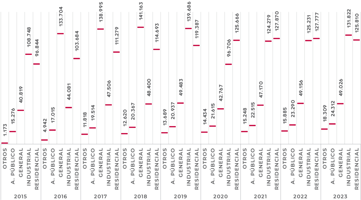
Gráfico 27: Chuquisaca: Evolución de las ventas de electricidad a consumidor final por categoría, 2015-2023 (Consumo en megawatts /hora)
