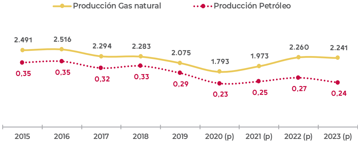
Gráfico 29: Producción de gas natural y petróleo, 2015-2023 (En millones de metros cúbicos)
