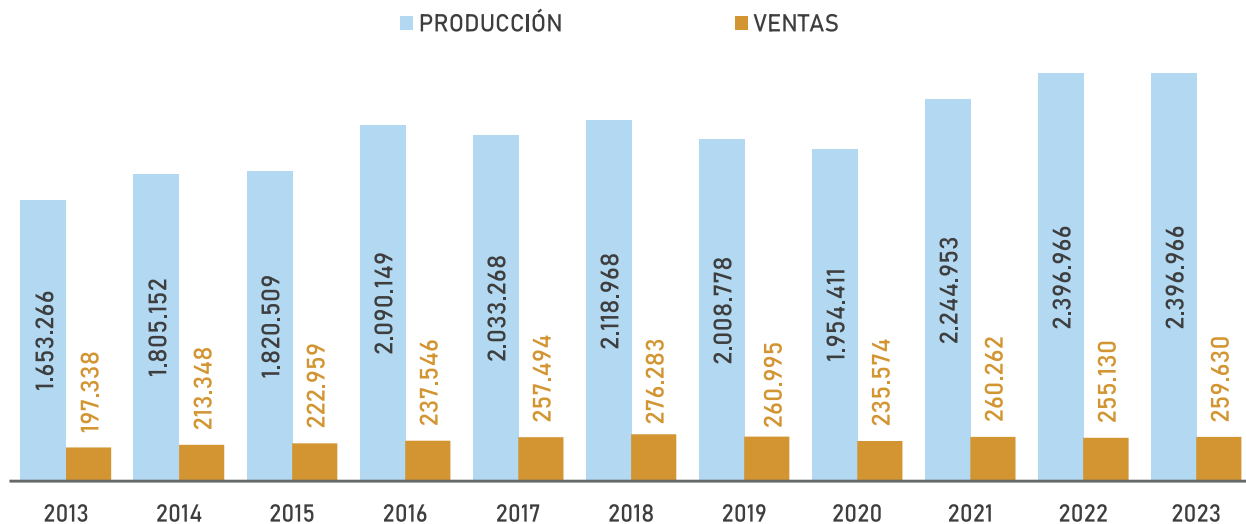
Gráfico 32: Producción y ventas de harina solvente de soya 2013 a 2023 (en toneladas)
