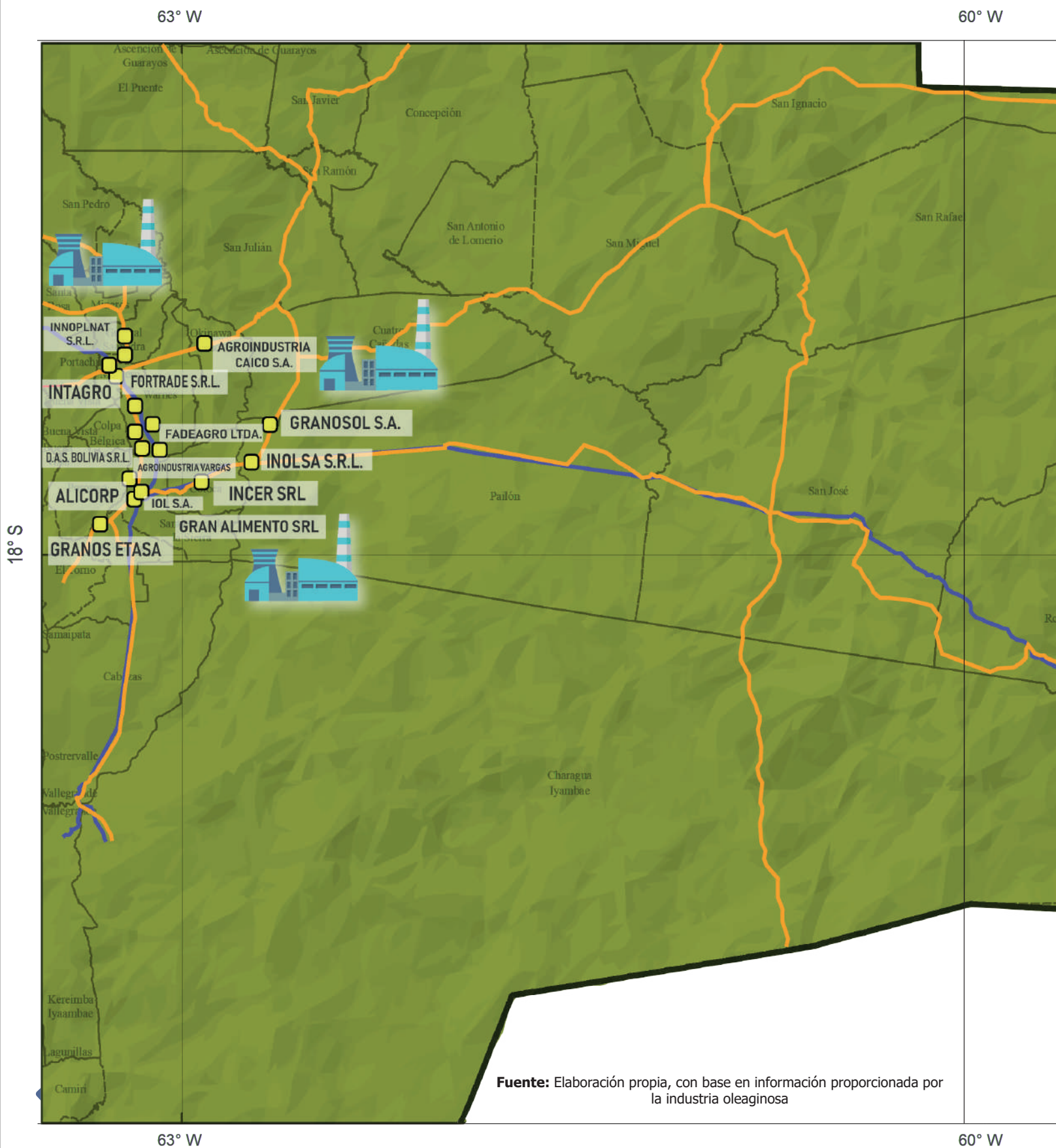
Mapa 10: Ubicación de plantas de transformación de la industria oleaginosa - Santa Cruz
