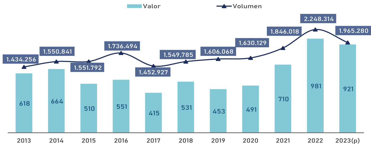
Gráfico 41: Exportación Harina Solvente 2013 - 2023 (en millones de dólares americanos y toneladas)
