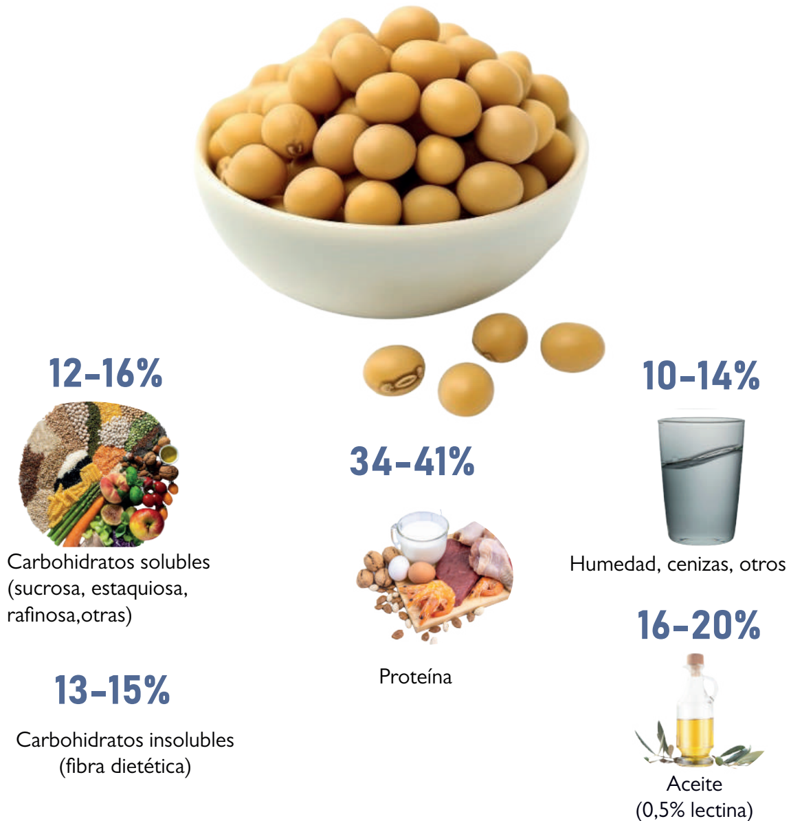
Gráfico 1: Composición del grano de soya
