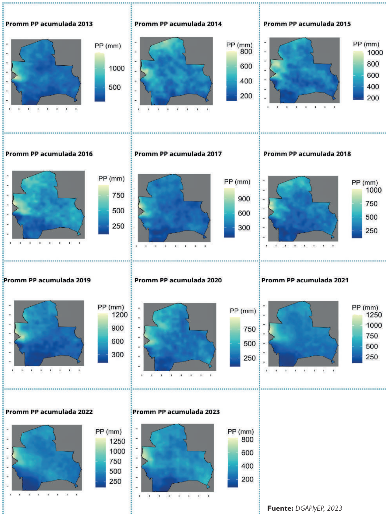
Mapa 3: Distribución espacio temporal de la precipitación acumulada 2013-2023
