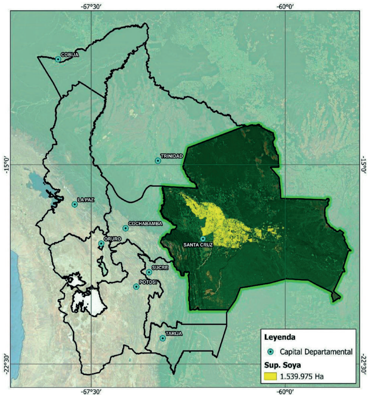
Mapa 7: Identificación de superficies de cultivos de Soya. Campaña Agrícola 2023
