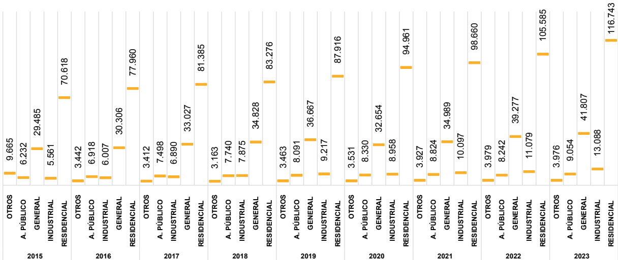
Gráfico 31: Evolución de las Ventas de Electricidad a Consumidor Final por Categoría (Consumo en Megawatts/hora)
