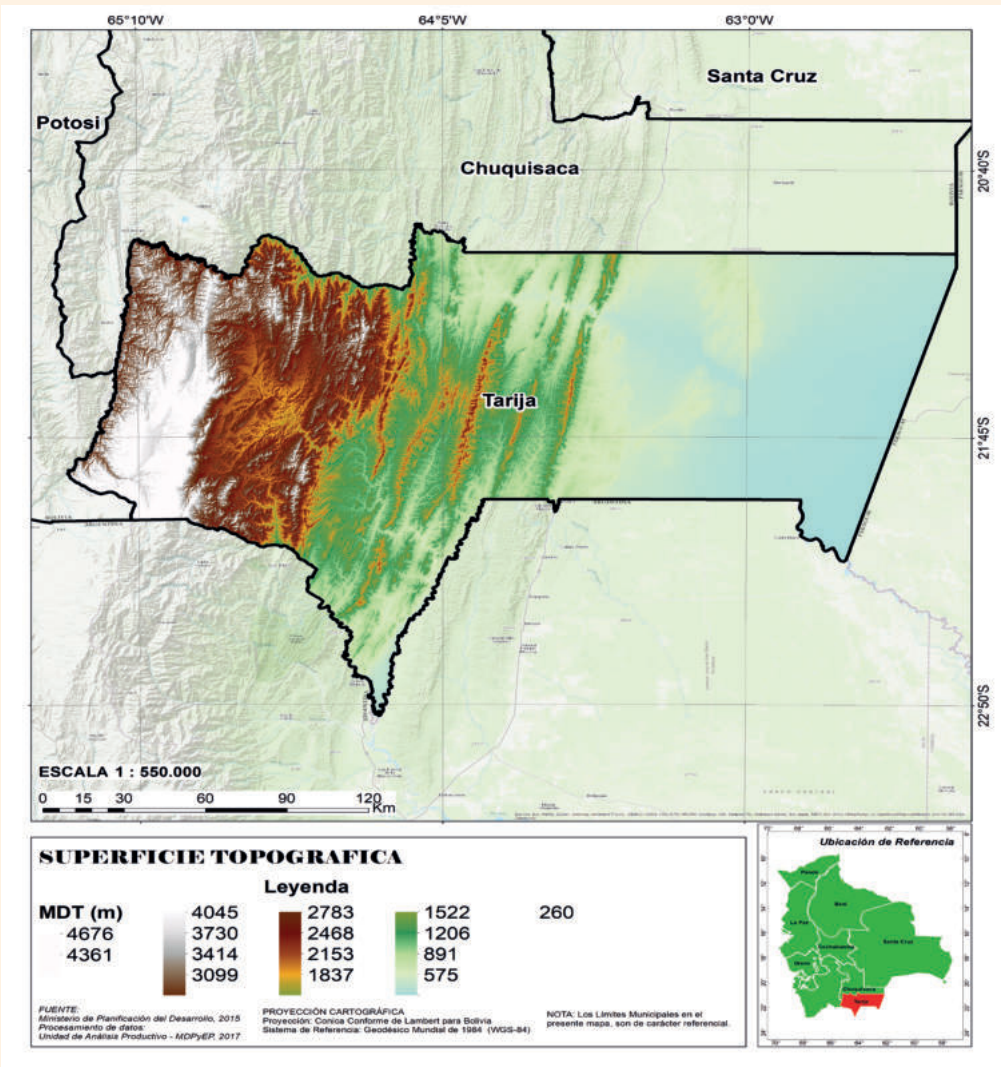
MAPA 1: SUPERFICIE TOPOGRÁFICA DEL DEPARTAMENTO DE TARIJA
