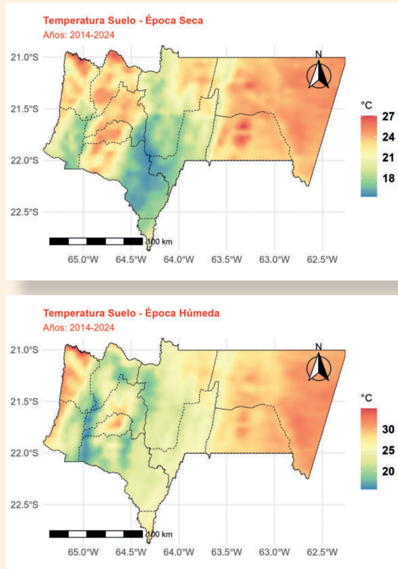
MAPA 3: TEMPERATURA PROMEDIO SUELO DEL DEPARTAMENTO DE TARIJA
