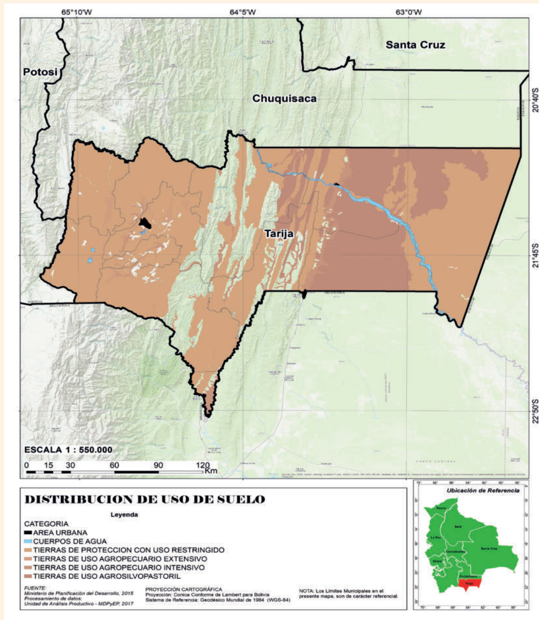
MAPA 2: DISTRIBUCIÓN DEL USO DE SUELOS DEL DEPARTAMENTO DE TARIJA
