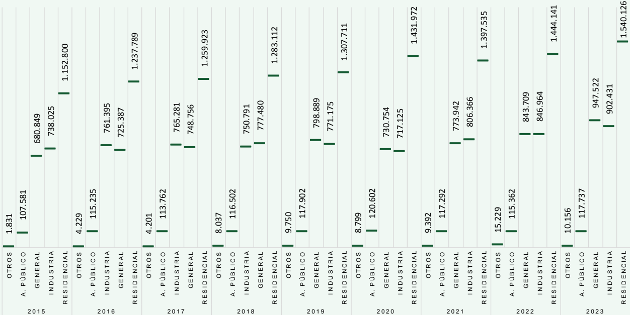
GRÁFICO 42: SANTA CRUZ, EVOLUCIÓN DE LAS VENTAS DE ELECTRICIDAD A CONSUMIDOR FINAL POR CATEGORÍA (CONSUMO EN MEGAWATTS / HORA)
