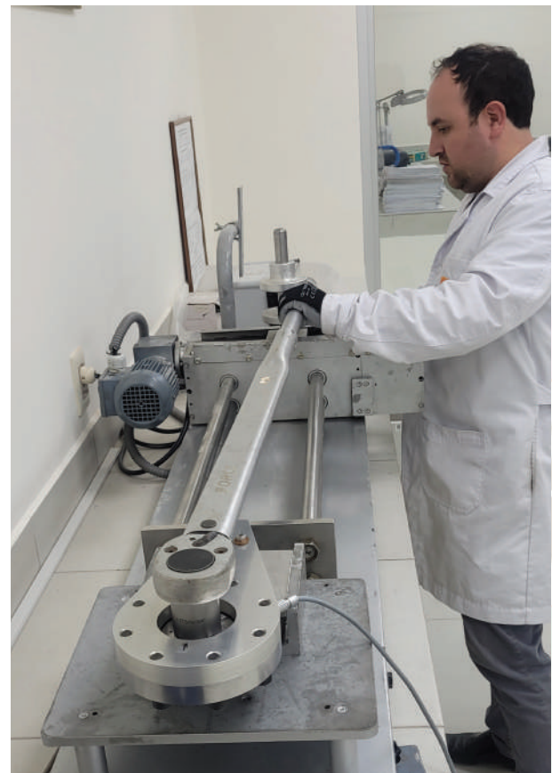
Bancada para medición de torque
