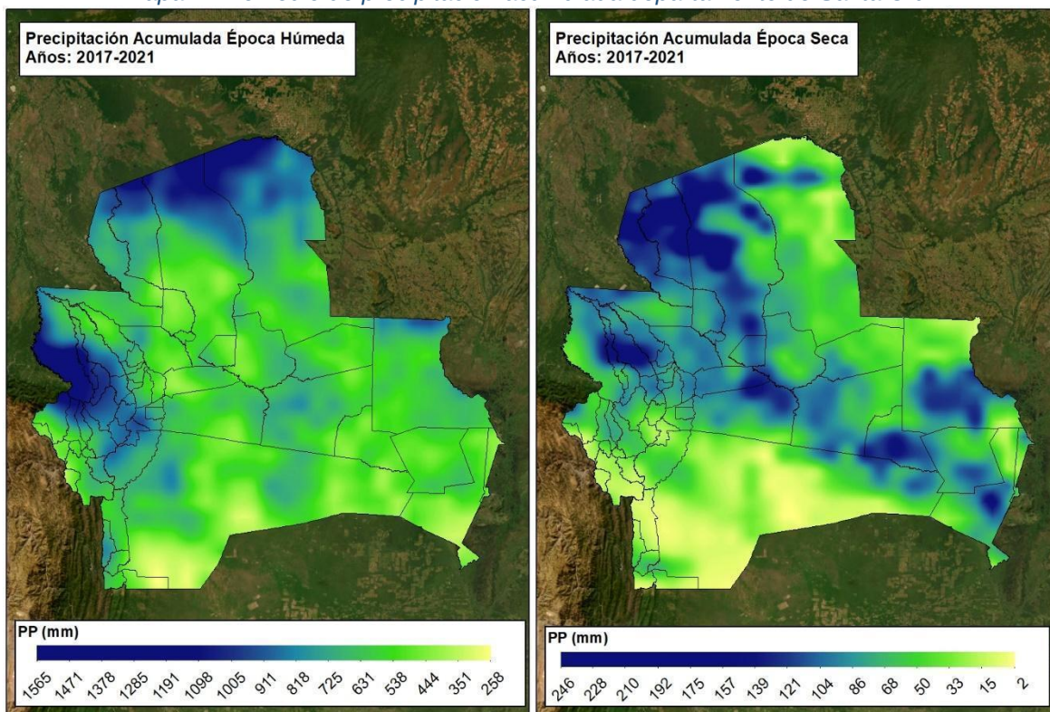
Mapa 4: Promedio de precipitación acumulada departamento de Santa Cruz
