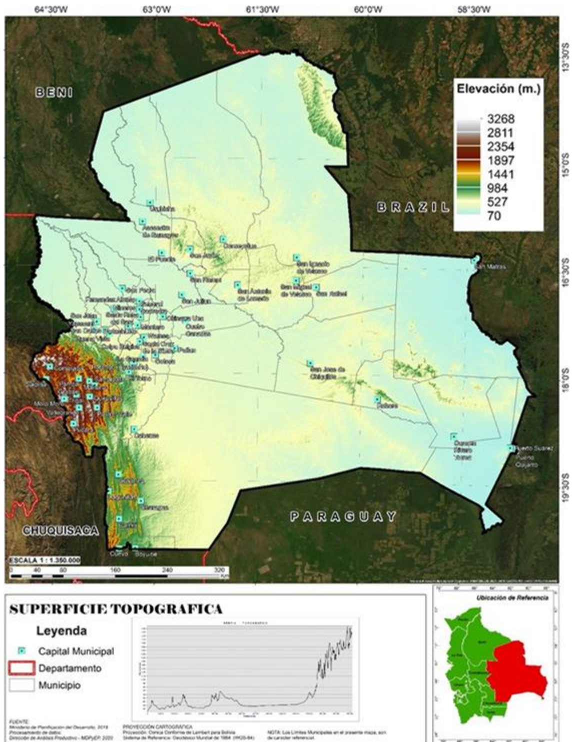
Mapa 1: Superficie Topográfica de Santa Cruz
